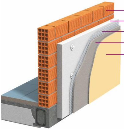
CAPPOTTO
